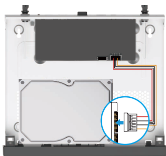
Toitekaabli ühendus
