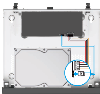
Andmesidekaabli ühendus
